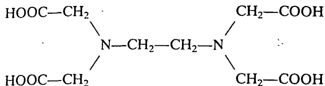
Figure 29.1 EDTA.
